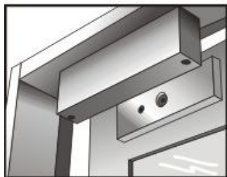
Instalación regular (puerta hacia-afuera)
