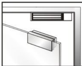
Con bracket tipo U para puertas de vidrio sin marco (opcional)
