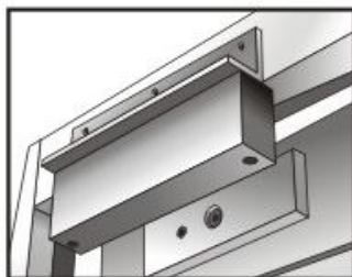
Con bracket tipo L para marcos angostos (opcional)
