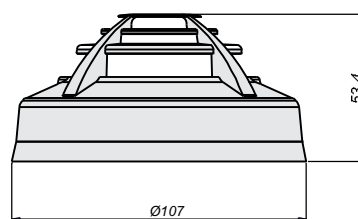
Montaje con zócalo bajo
