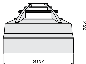
Montaje con zócalo alto
